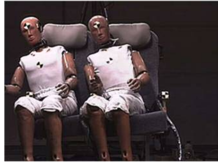
側面衝突模擬試験
